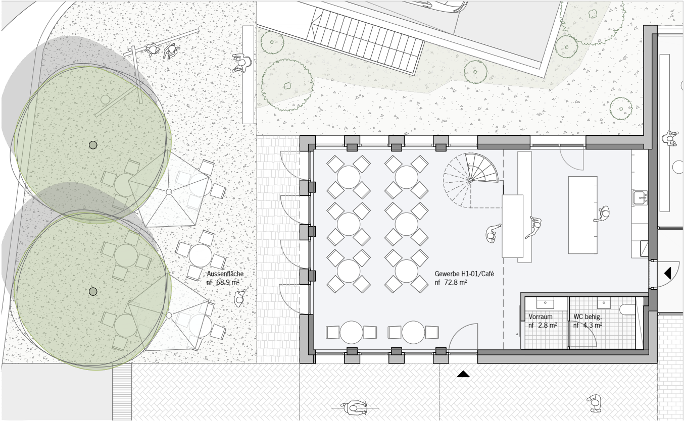
N0 (Erdgeschoss)
