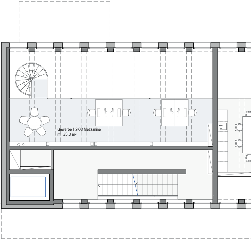
N0 - Erdgeschoss
